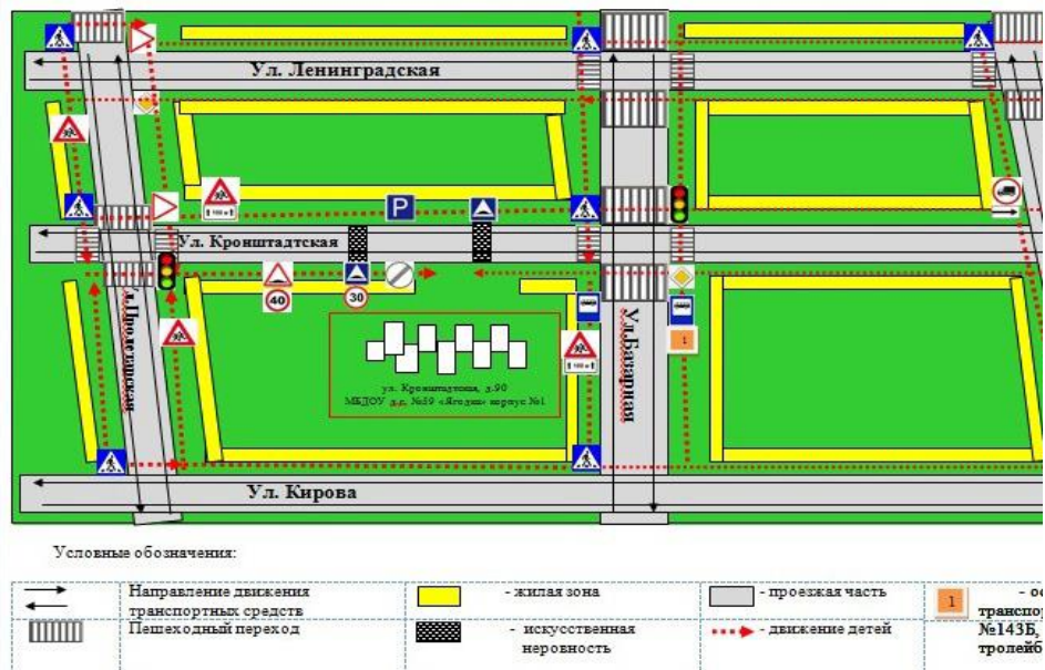
1.2. Схема организации дорожного движения в непосредственной близости от образовательного учреждения с размещением сопутствующих средств, маршруты движения детей и расположение парковочных мест автотранспорта Корпус № 1 МБДОУ "Детский сад № 59 "Ягодка"
