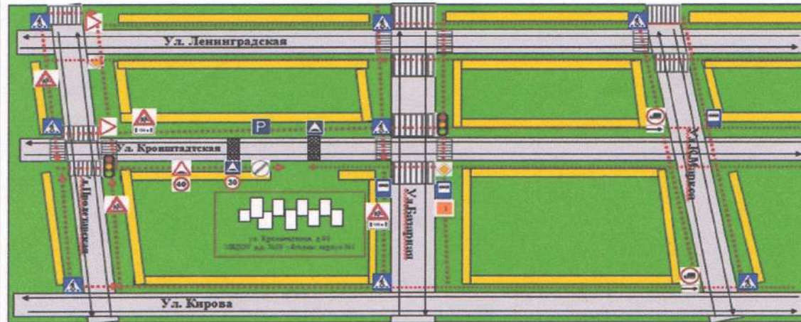
1.2. Схема организации дорожного движения в непосредственной близости от образовательного учреждения с размещением сопутствующих технических средств, маршруты движения детей и расположение парковочных мест автотранспорта Корпус № 1 МБДОУ "Детский сад № 59 "Ягодка"
